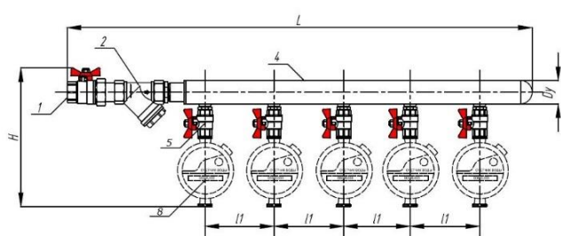
Коллекторный узел ХВС и ГВС без регулятора, со счетчиками (Вариант 6)
