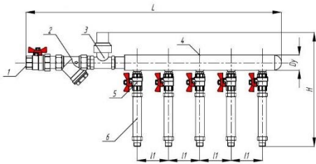
Коллекторный узел ХВС и ГВС с общим регулятором (Вариант 1)
