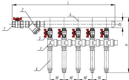
Коллекторный узел ХВС и ГВС с индивидуальным регулятором (Вариант 3)
