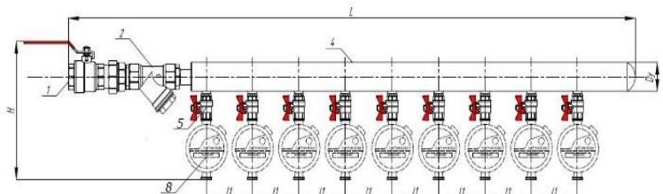
Коллекторный узел ХВС и ГВС без регулятора, со счетчиками (Вариант 6)
