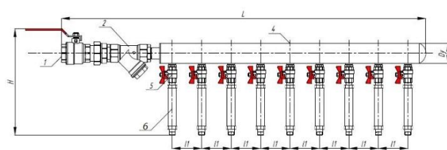
Коллекторный узел ХВС и ГВС без регулятора (Вариант 5)
