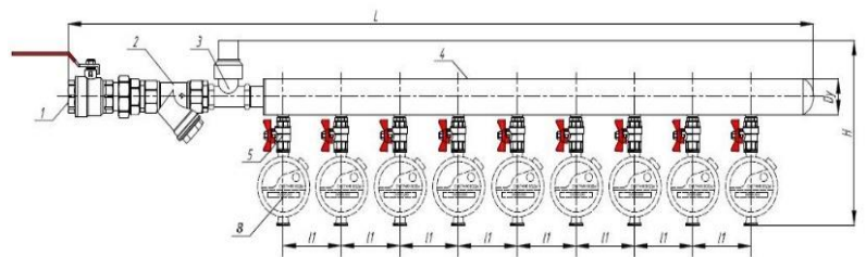
Коллекторный узел ХВС и ГВС с общим регулятором и счетчиками (Вариант 2)
