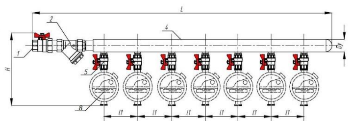
Коллекторный узел ХВС и ГВС без регулятора, со счетчиками (Вариант 6)
