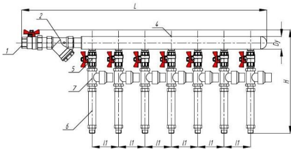
Коллекторный узел ХВС и ГВС с индивидуальным регулятором (Вариант 3)
