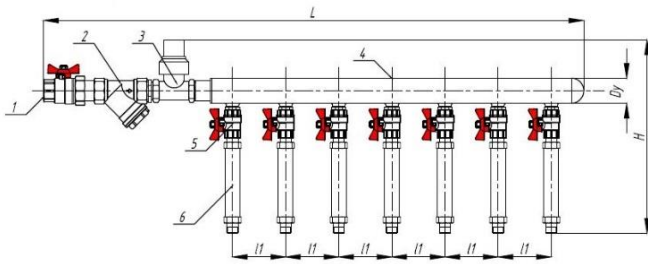
Коллекторный узел ХВС и ГВС с общим регулятором (Вариант 1)
