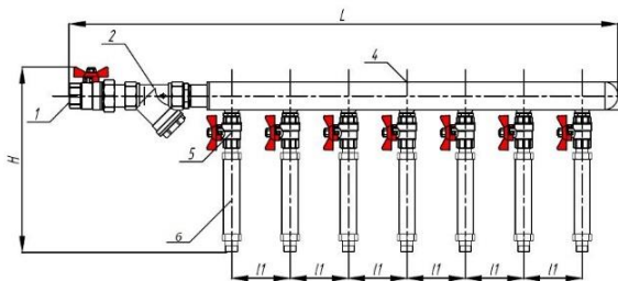
Коллекторный узел ХВС и ГВС без регулятора (Вариант 5)
